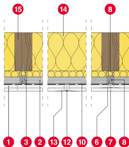
Przekrój pionowy
