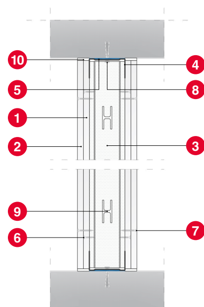
Przekrój pionowy
