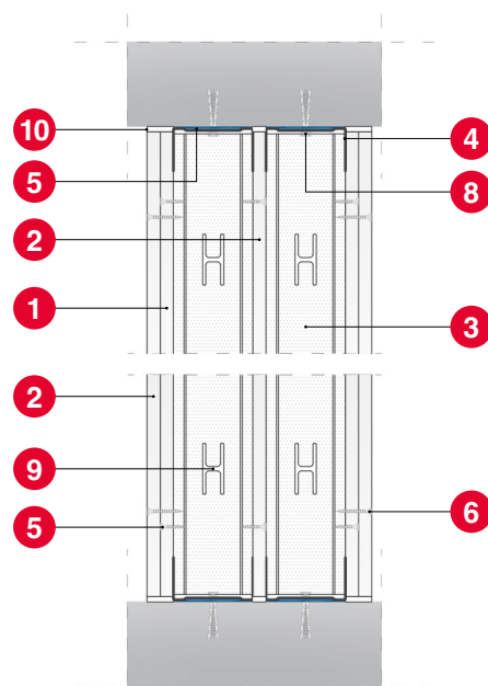
Przekrój pionowy
