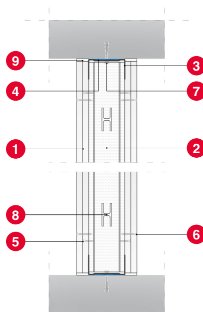
Przekrój pionowy
