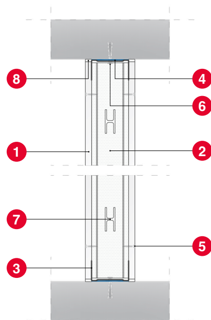
Przekrój pionowy
