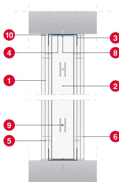
Przekrój pionowy
