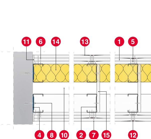
Przekrój poziomy
