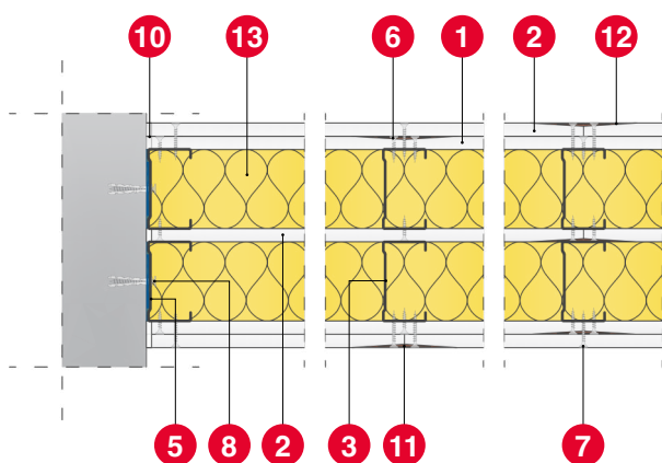
Przekrój poziomy
