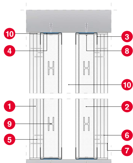
Przekrój pionowy
